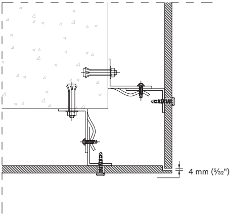
PILASTER EDGE
