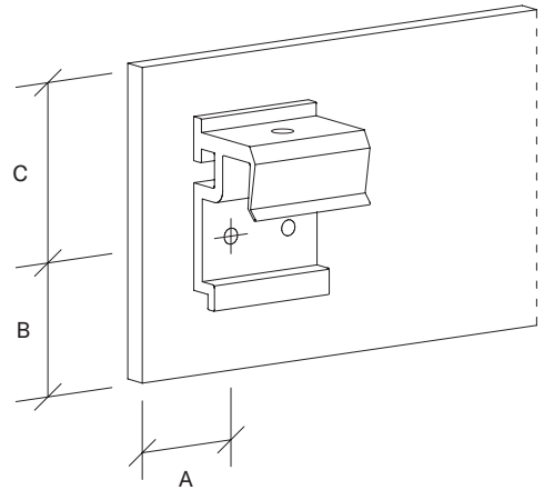
A. Lateral edge distance: 24 mm ( \frac{15}{16} ") B. Bottom edge distance: 45 mm ( 1 \frac{4}{64} ") C. Upper edge distance: 58 mm ( 2 \frac{5}{32} ")
